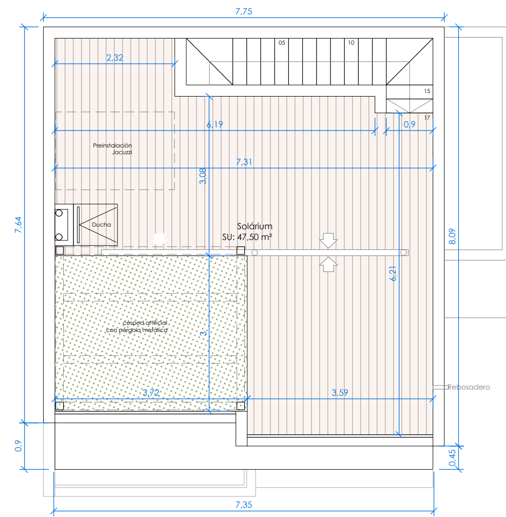
PLANTA CUBIERTA
