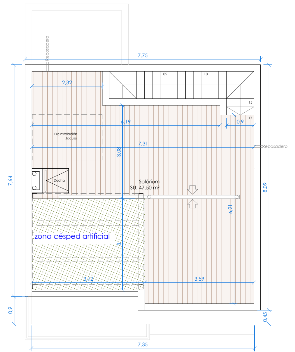
PLANTA CUBIERTA
