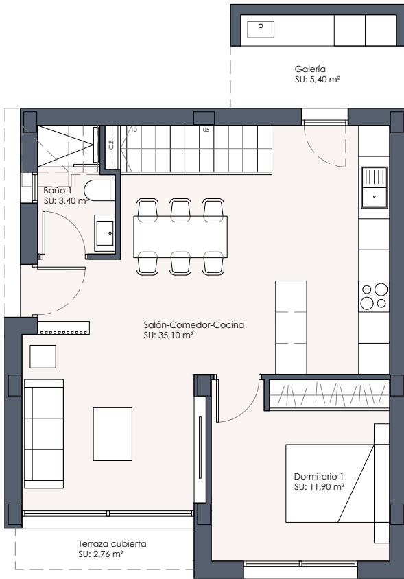
PLANTA BAJA
