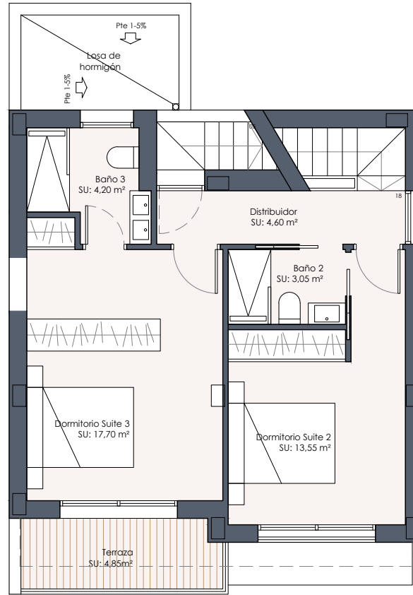
PLANTA PRIMERA
